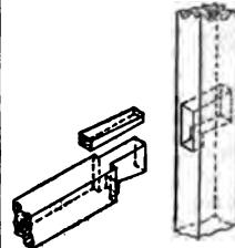
FIG. 15.—Dovetailed Tenon.
