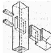
FIG. 13.—Mortice and Tenon.
