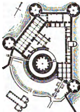
FIG. 7.—Coucy: Plan.
