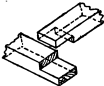
FIG. 10.—Halving.
