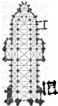
FIG. 6.—Plan of Sens Cathedral.
