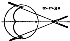
FIG. 6. a > 1/2 a
