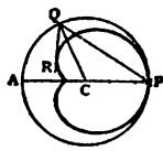
FIG. 1. c = a
